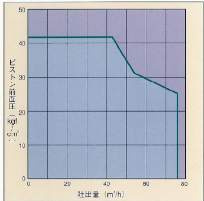
■圧送性能線図
